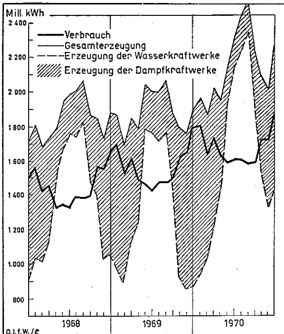
Stromerzeugung und Stromverbrauch (Linearer Maßstab; Mill. kWh)
